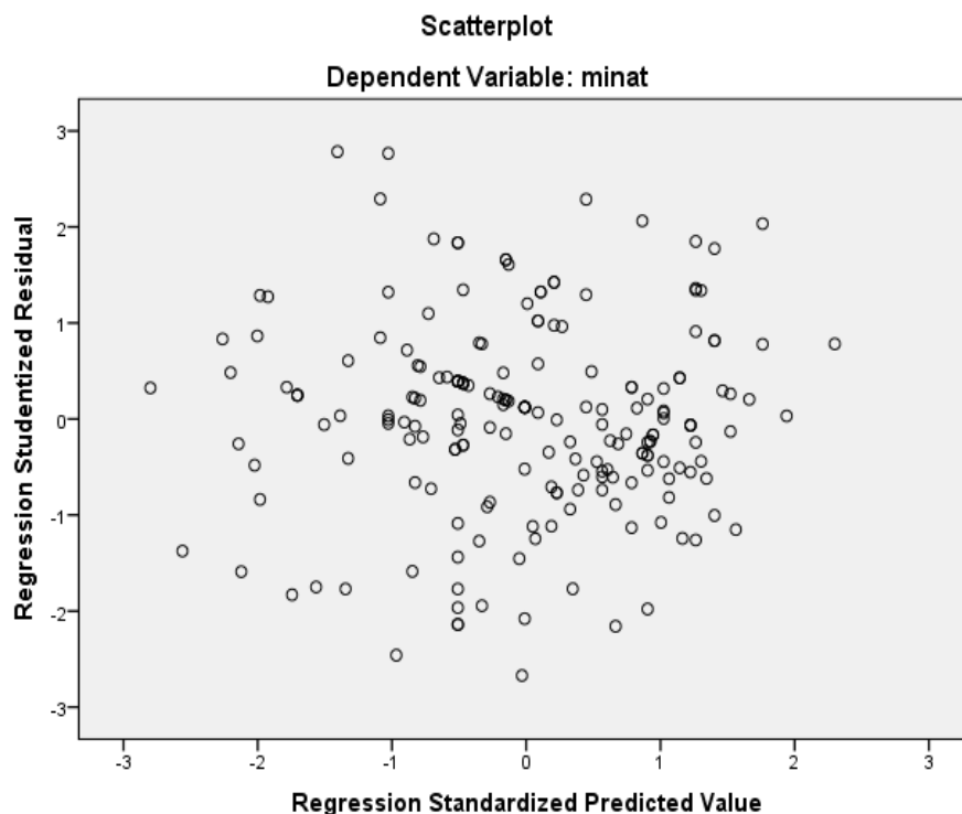
Gambar 4 Uji Heteroskedastisitas
